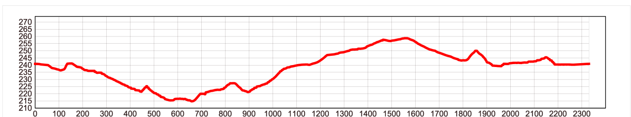
Lengdeprofil starter ved utgang standplass
